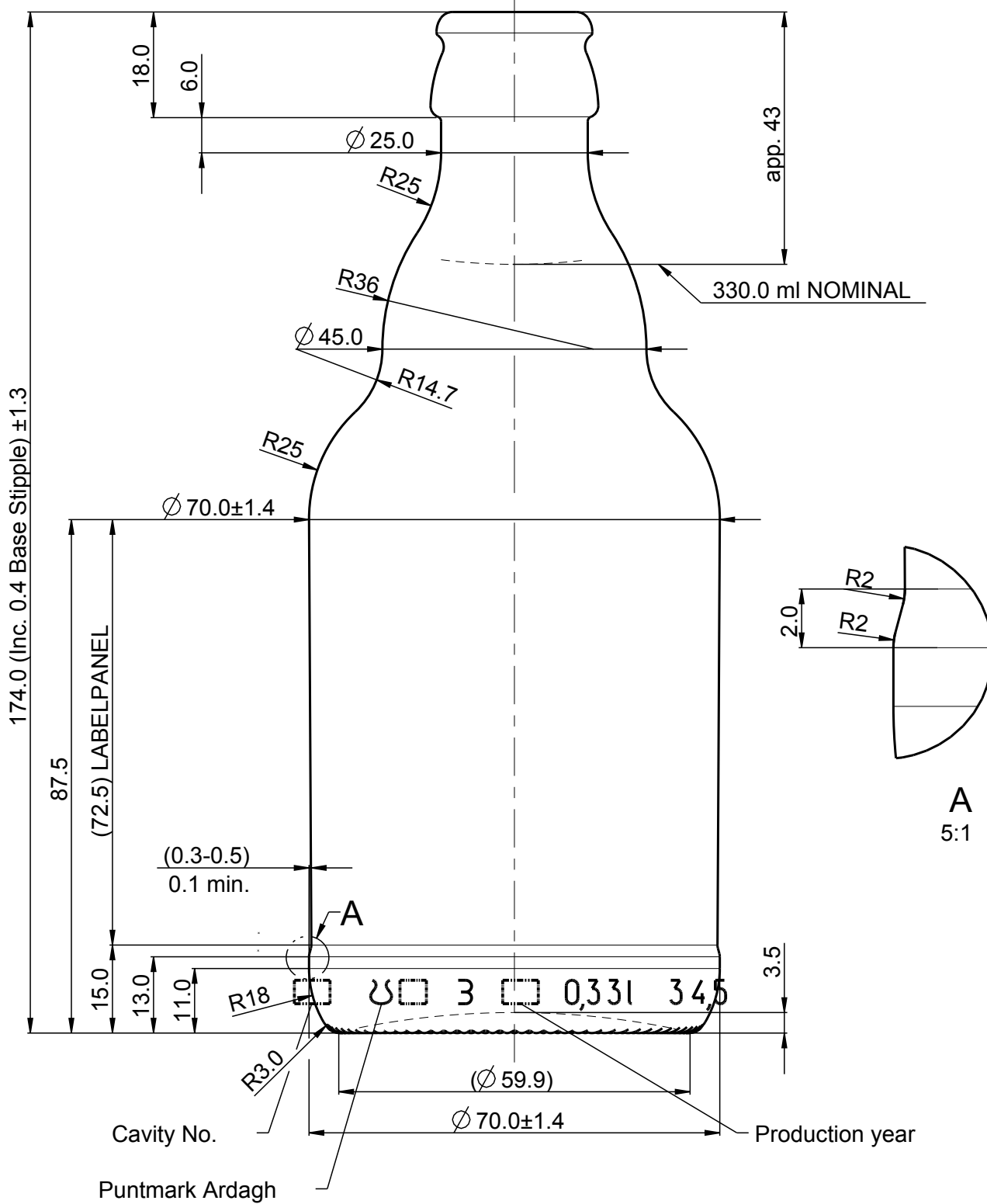
Front view 26H 180 Crown Cork DIN EN 14634:2005-01
